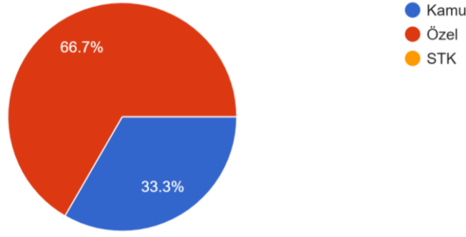
Şekil 1. Çalışılan iş yeri
