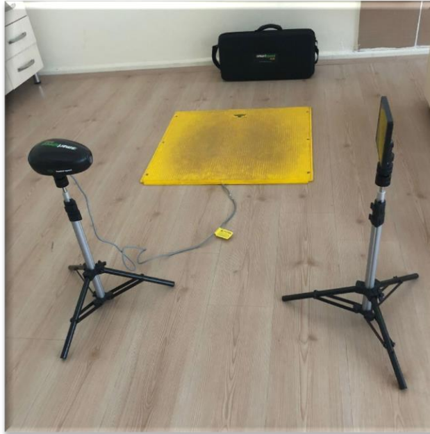
Resim- 9. Smart speed fotosel bağlantılı dikey sıçrama pedi
