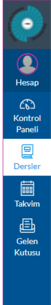
Menü çubuęu
